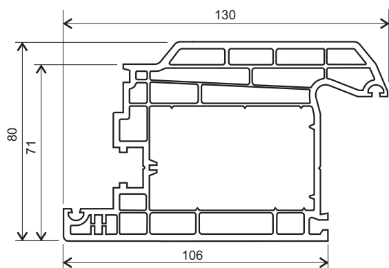
křídlo dveří otvíravých dovnitř
