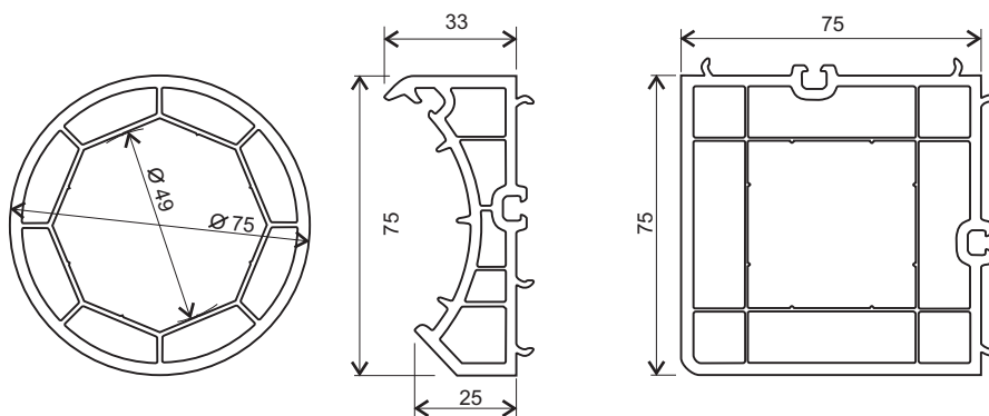
variabilní roh
