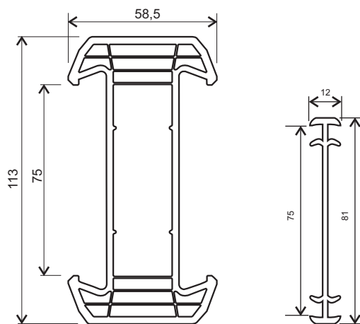
spojovací profil
