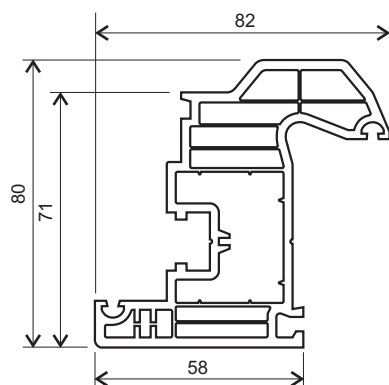
křídlo okenní
