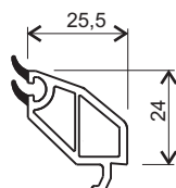
zasklívací lišta
