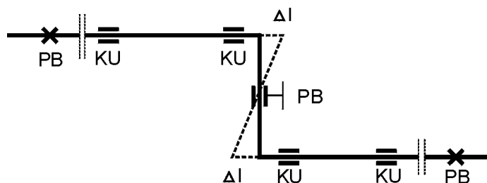
obr. č. 7 Kompenzátor tvaru - Z
