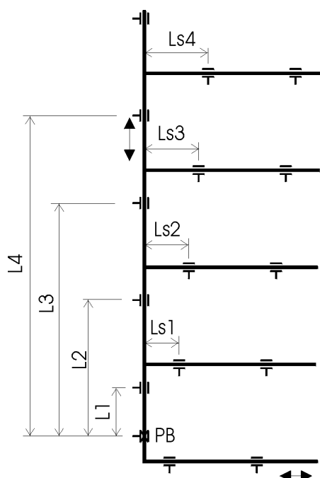
obr. č. 13 Pevný bod ve spodní části stoupačky
