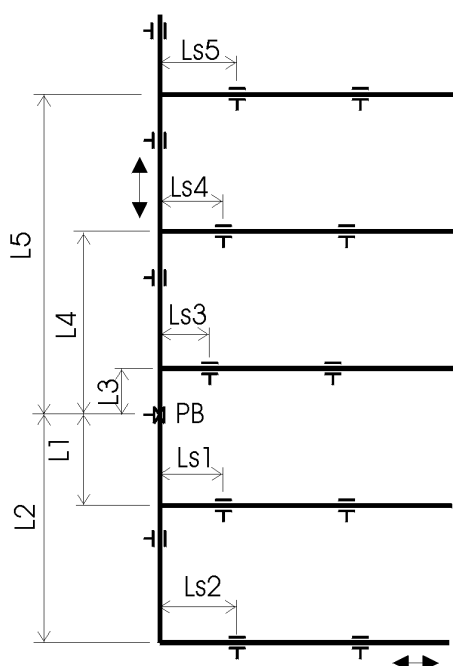
obr. č. 14 Pevný bod ve střední části stoupačky
